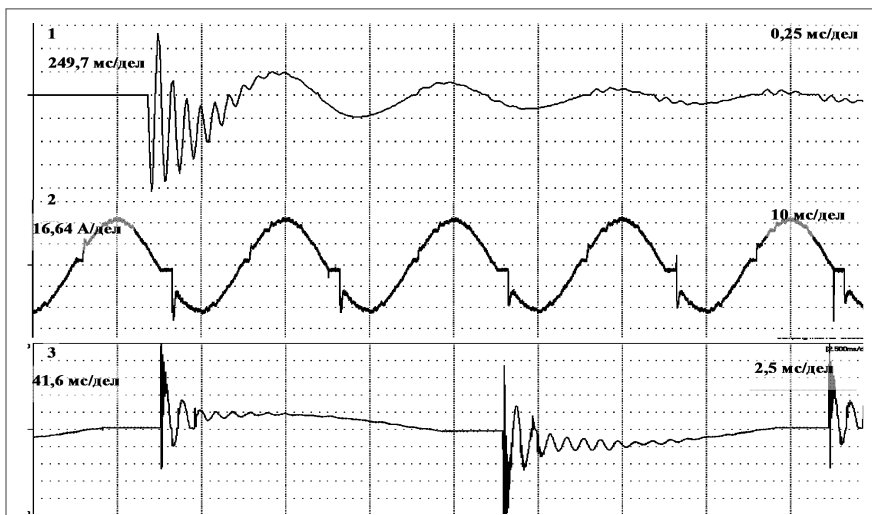
Рис. 2. Экспериментальные осциллограммы тока дуги в сети 10 кВ при I_R = 2,5I_C для режима перемежающейся (1, 3) и устойчиво горящей (2) дуги
